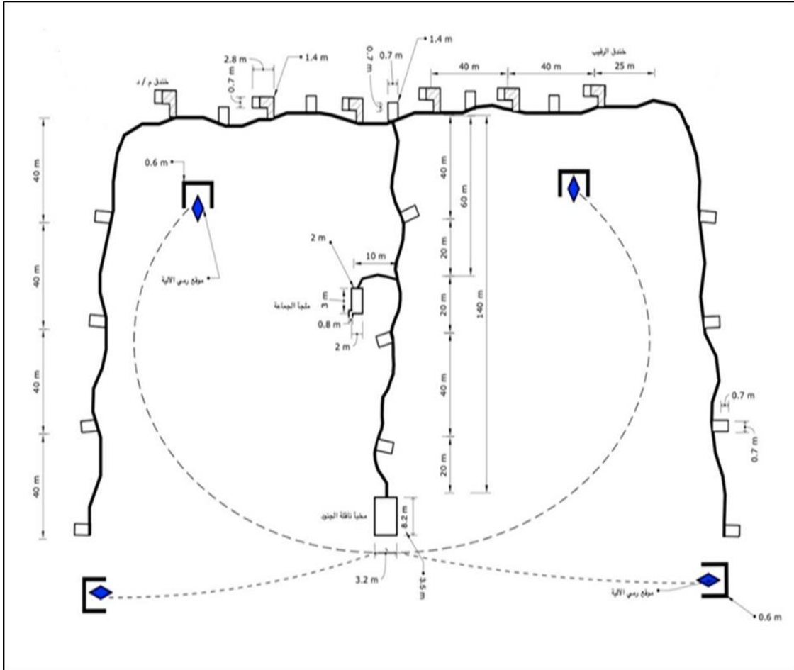
الشكل رقم (49) مثال على موقع دفاعي لجماعة العمق
