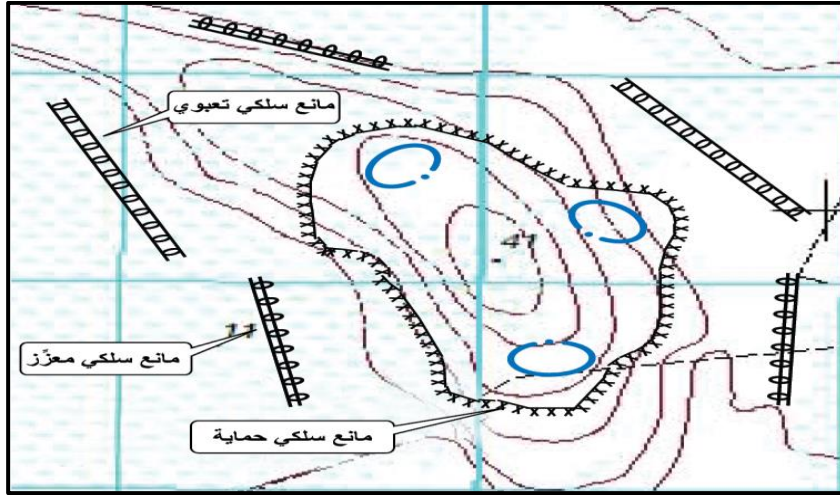
الشكل رقم (40) مثال على الأنواع الثلاثة من الموانع السلكية
