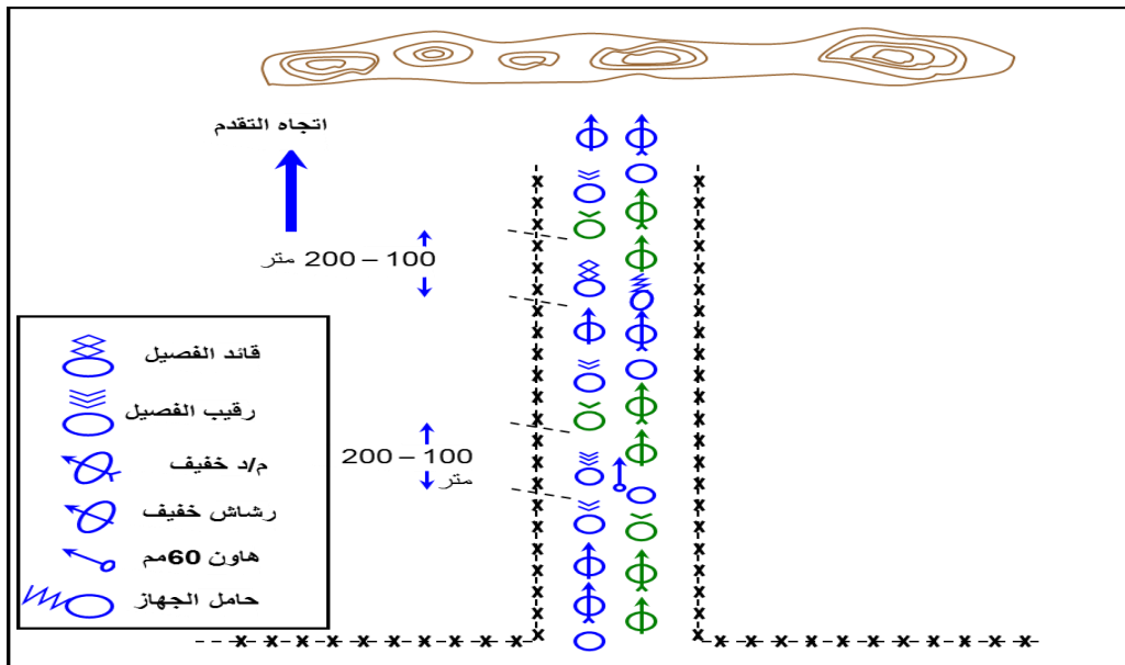
الشكل رقم (9) تشكيل الخط المزدوج بمحاذاة سياج شائك
