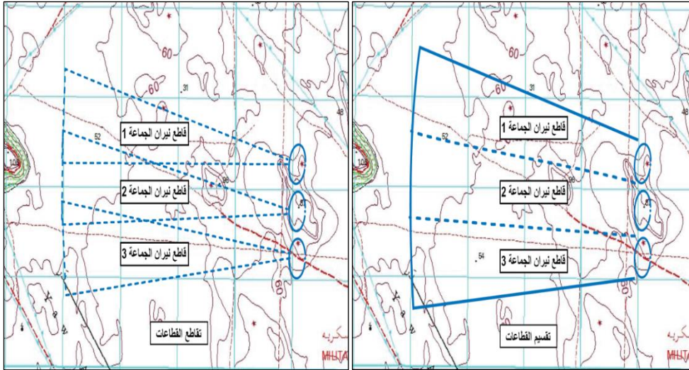
الشكل رقم (30) تقاطع وتقسيم قطاعات الرمي
