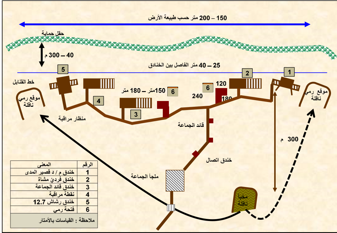
الشكل رقم (48) مخطط خنادق وملجأ جماعة
