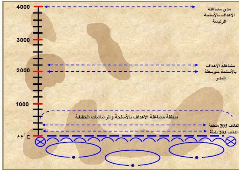
الشكل رقم (29) خطوط اشتباك الأسلحة حسب المدى
