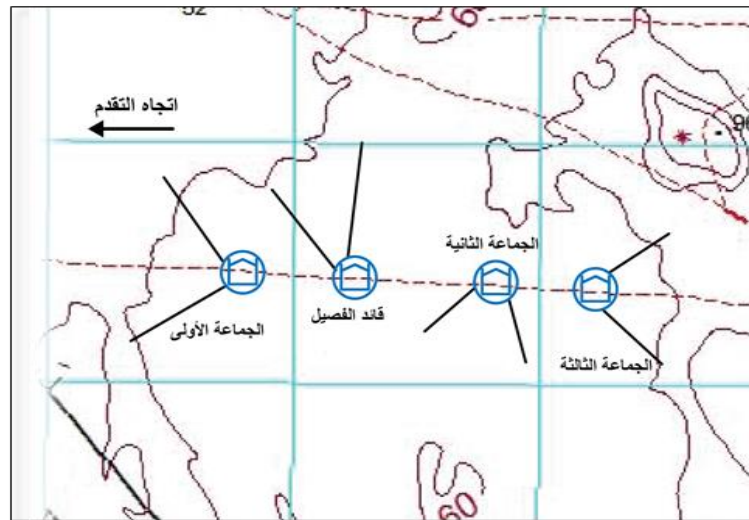
الشكل رقم (17) تشكيلة الخط المنفرد
