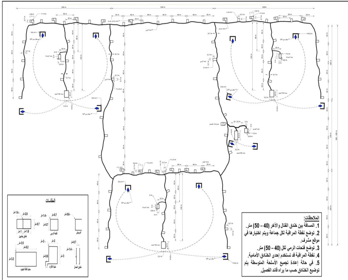
الشكل رقم (50) مثال على موقع دفاعي لفصيل مشاة آلي
