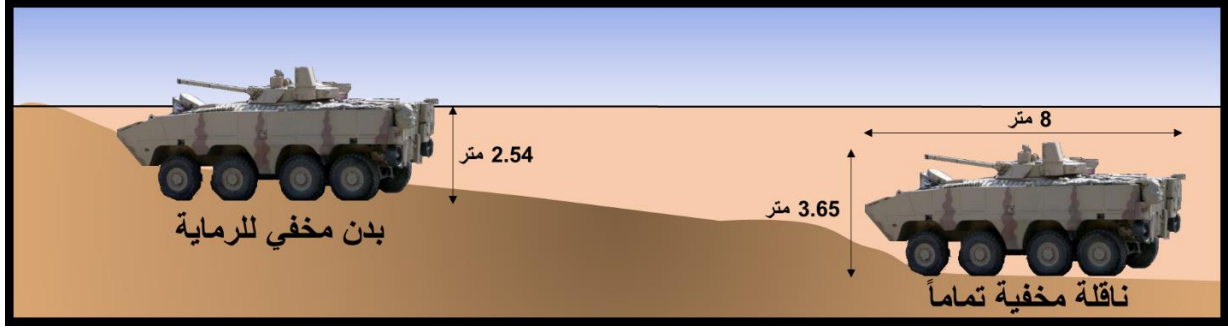
الشكل رقم (43) موقع قتالي لآلية
